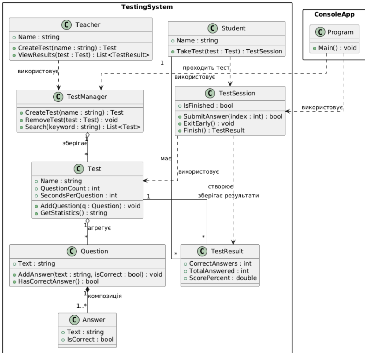
Діаграма класів: Система тестування
